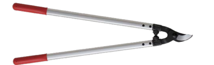
LPB-20L 1/10 EAN 4965280448316 Loppers 772 mm, red/grey B C 772 1055 LPB-20-1 / LPB-20-2 34
